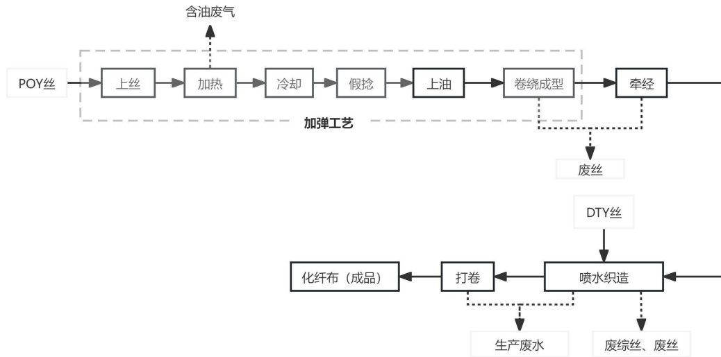
图 3-4 本项目各类纺织面料生产工艺及产污流程图
