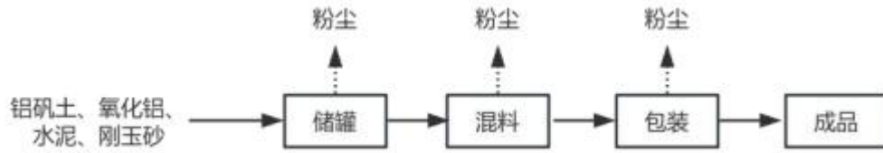
图 3-5 本项目不定型耐火材料生产工艺及产污流程图
