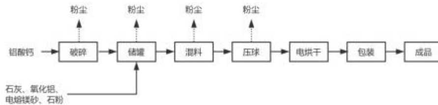
图 3-4 本项目合成渣生产工艺及产污流程图
