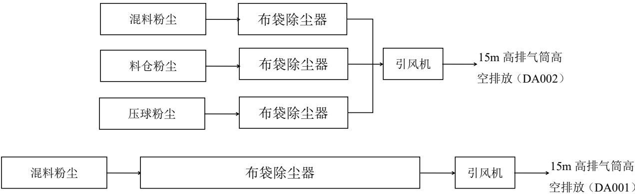
图 4-2 本项目废气处理工艺流程
